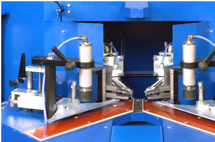
Détails des butées et des poinçons
