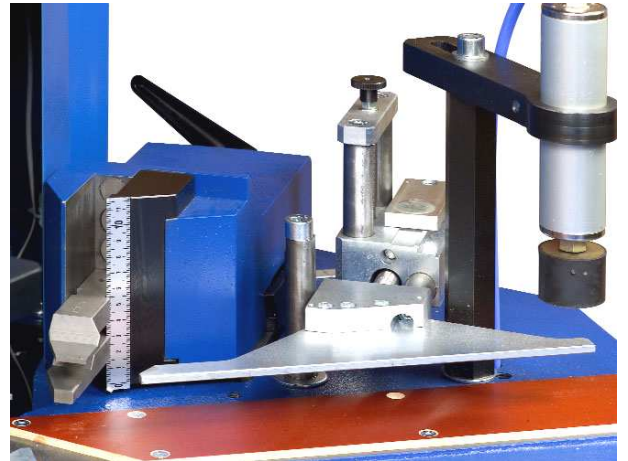
Détails des butées et des poinçons
